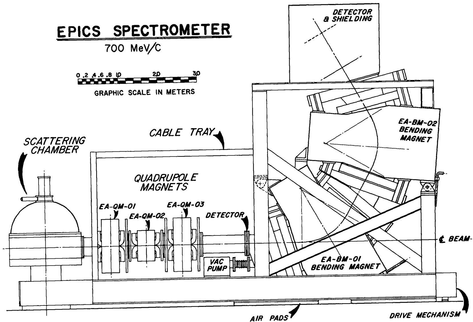
Fig. 17. EPICS Spectrometer.
