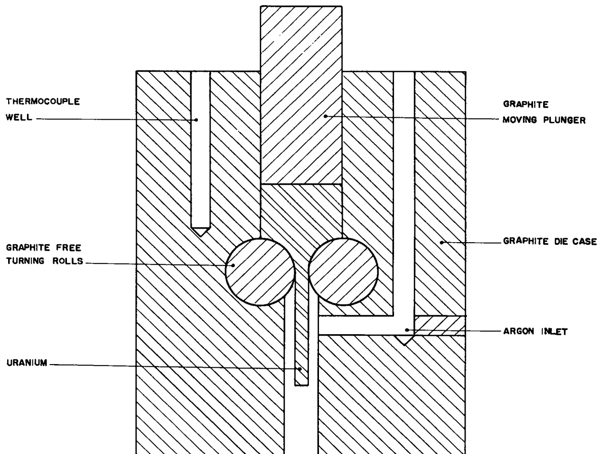
ROLLING DIE ASSEMBLY
