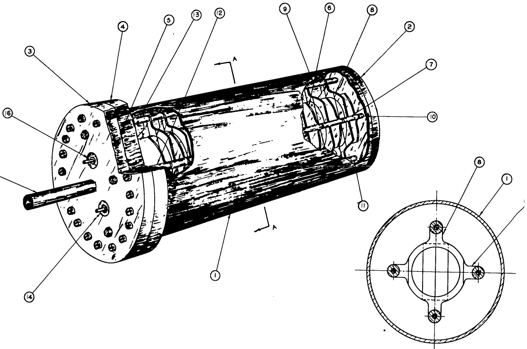
SECTION A-A
